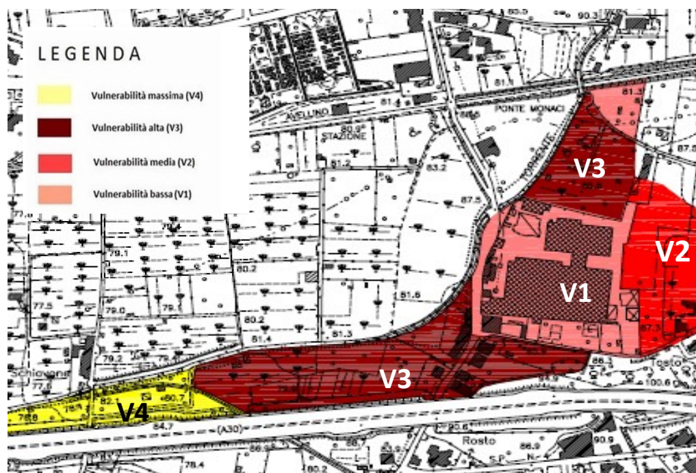
Comune di Mercato San Severino (SA) – Torrente Solofrana – Piano Stralcio di Assetto idrogeologico dell'ex Autorità di Bacino Regionale Campania Centrale – Stralcio Mappa della Vulnerabilità idraulica vigente Tavola Vuln-467013
