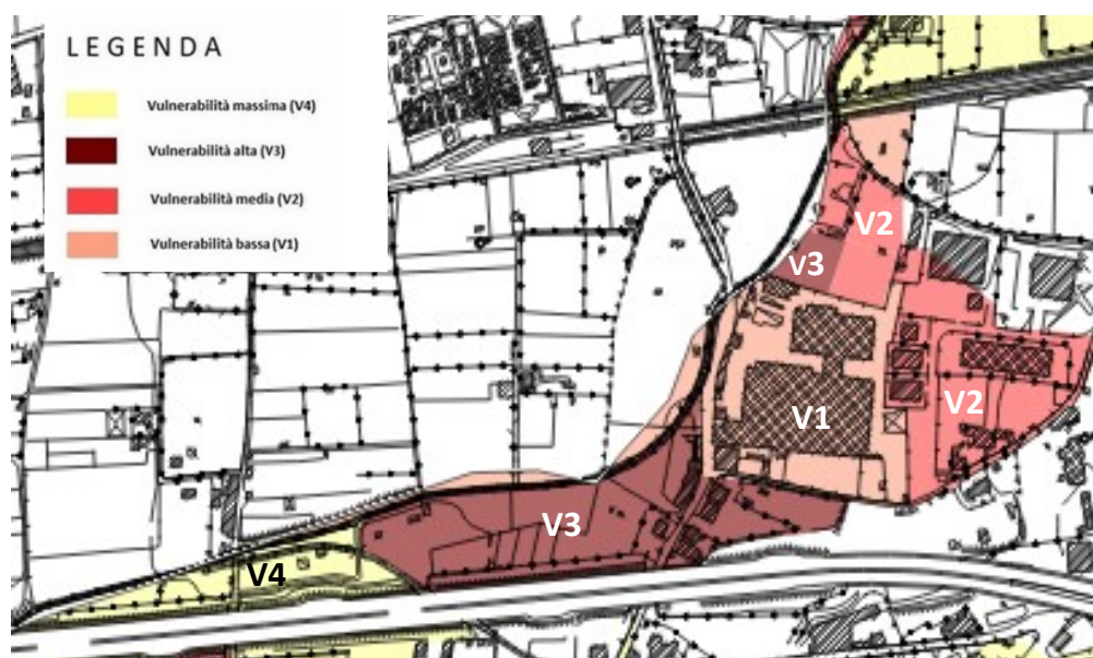
Comune di Mercato San Severino (SA) – Torrente Solofrana – Piano Stralcio di Assetto idrogeologico dell'ex Autorità di Bacino Regionale Campania Centrale – Stralcio Mappa della Vulnerabilità idraulica proposta Tavola Vuln-467013
